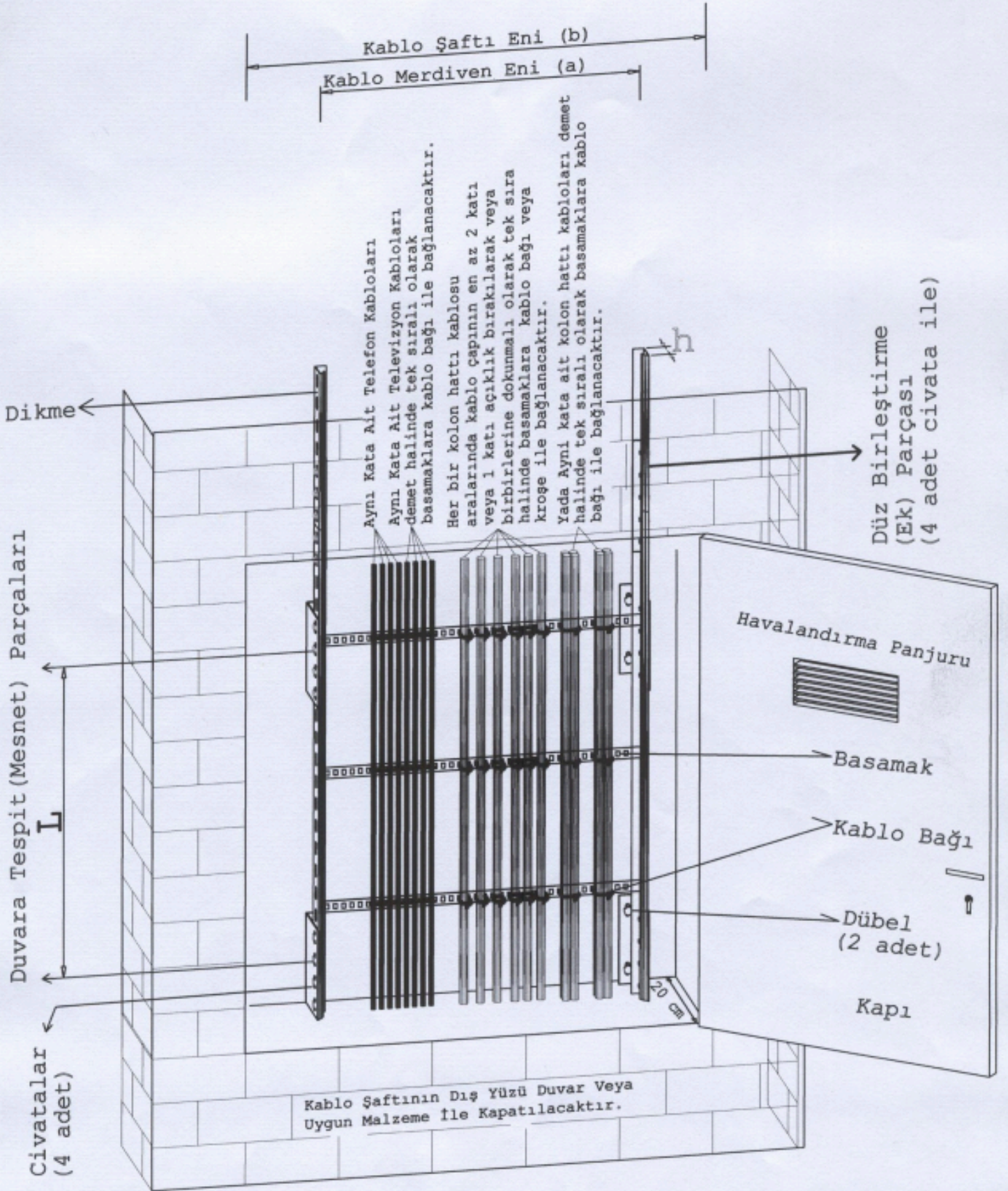
Şekil 1- Kablo Şaftı ve Örnek Kablo Merdiveni
